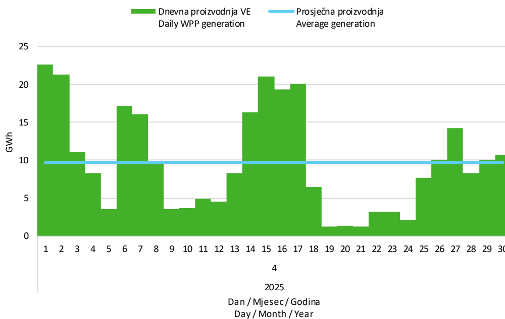
Slika 5 Dnevna proizvodnja svih vjetroelektrana u travnju 2025. godine
