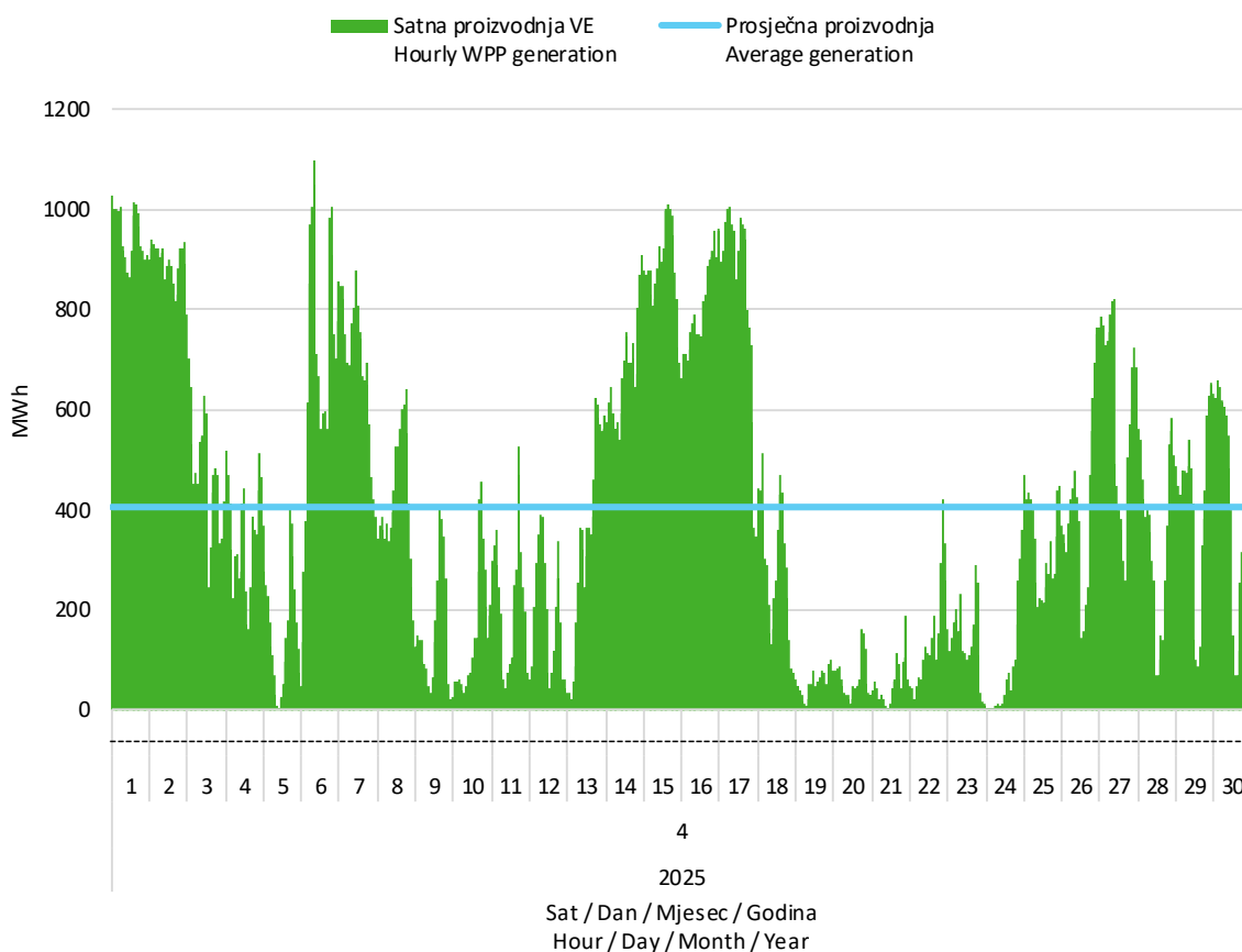
Slika 2 Satna proizvodnja svih vjetroelektrana u travnju 2025. godine
